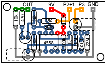
参考:裏面
