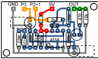
配置図
